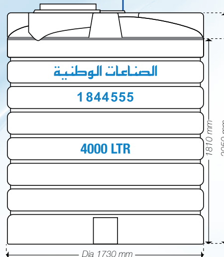
أبعاد الخزان Tank Dimensions
